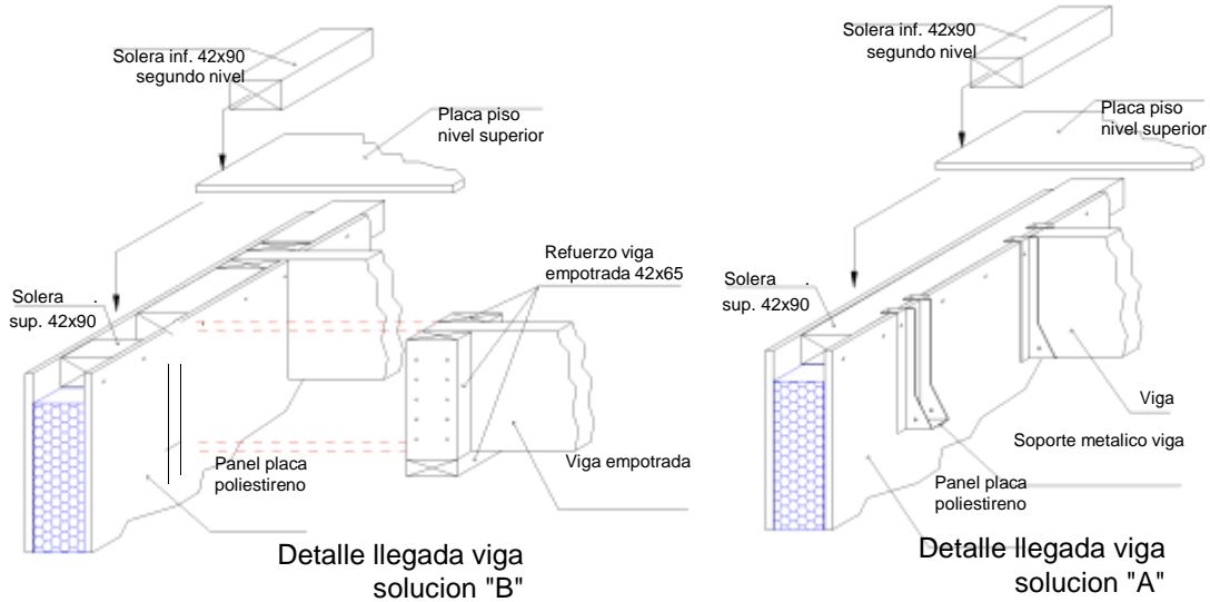
Fig. 5 Llegada viga-panel.
