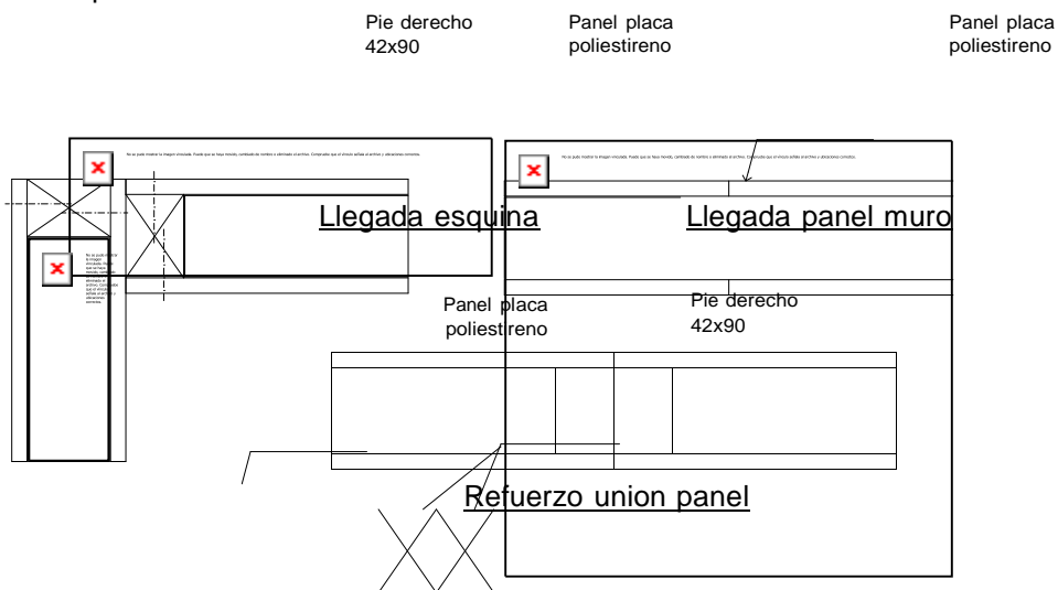
Fig. 4 Unión paneles.
